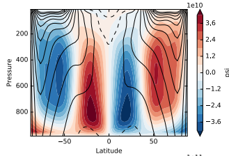
Streamfunction
