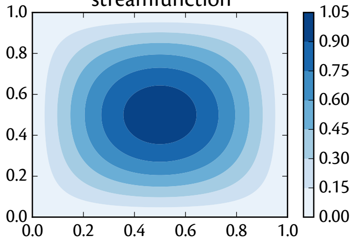
streamfunction
